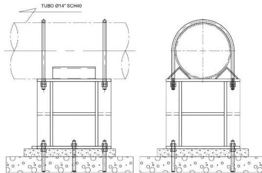
SOPORTE TÍPICO S1
