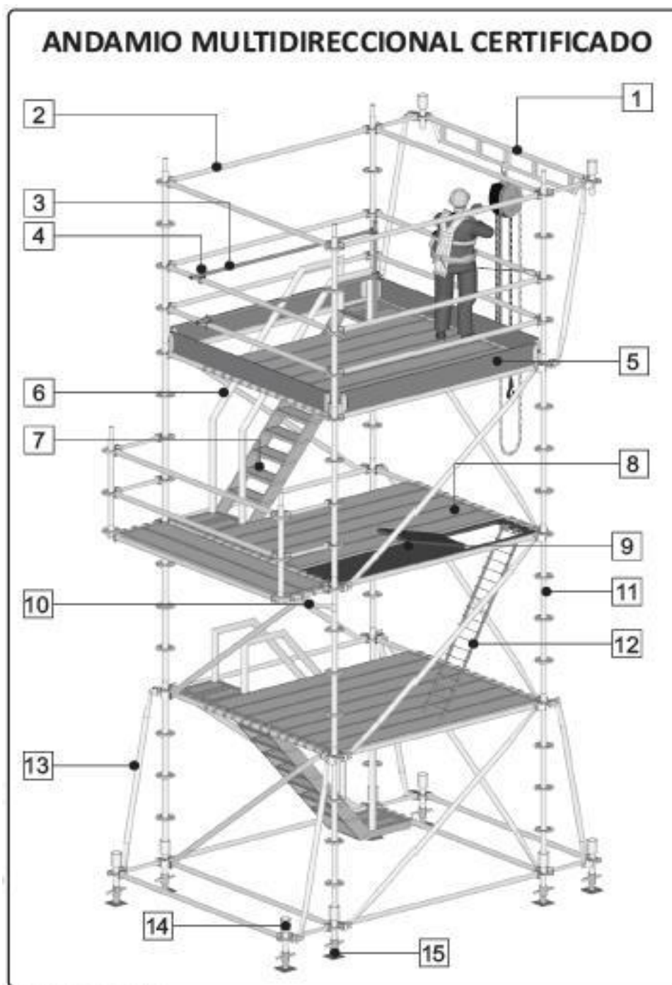
Ilustración 1. Esquema de andamio multidireccional certificado.
