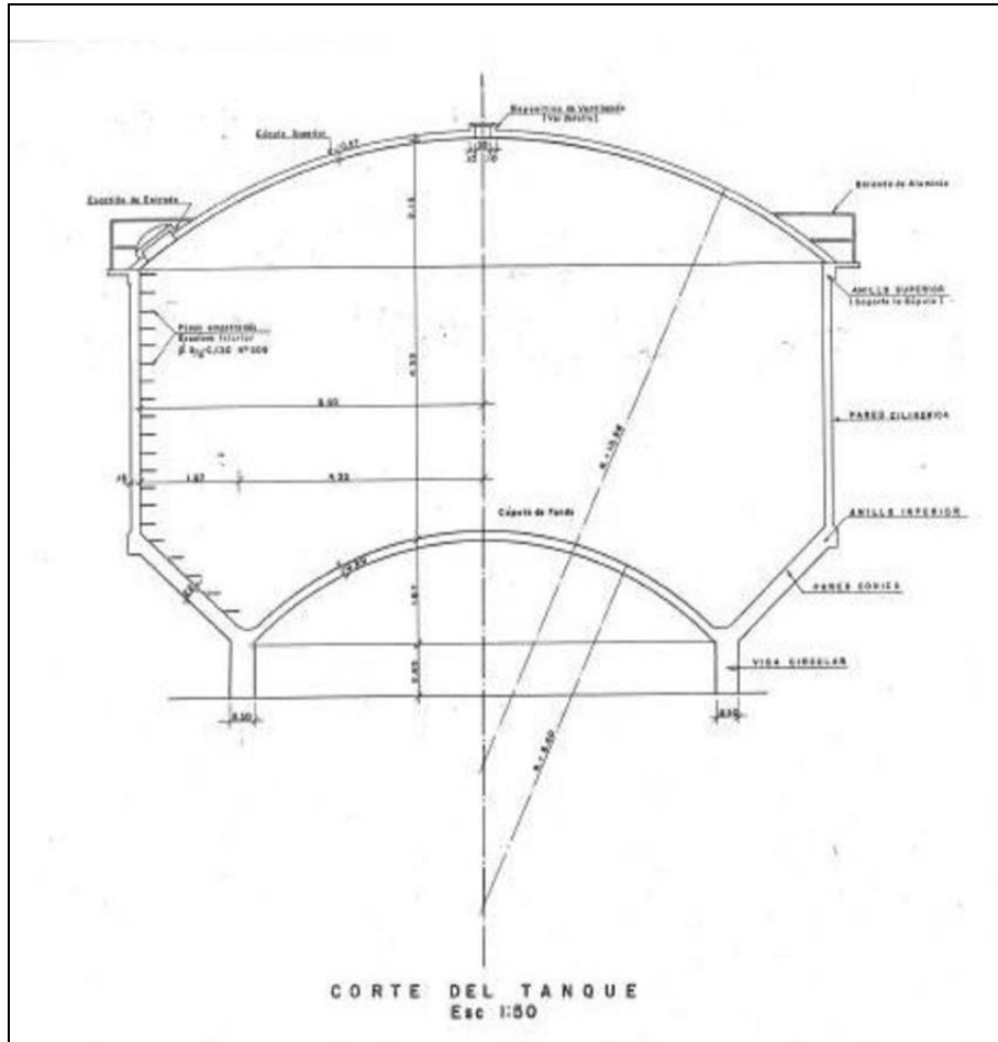
Esquema 2: Corte de Tanque elevado Loma sede loma.
